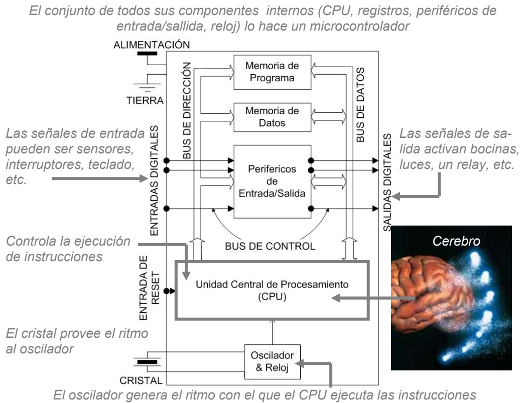
Figura 73. Diagrama de Bloques de un Microcontrolador. Cuando en un mismo integrado se encuentran unidos el CPU, memoria, oscilador, registros de entrada/salida, se dice que es un microcontrolador. El CPU, es el cerebro o la parte del microcontrolador que controla la ejecución de instrucciones.
