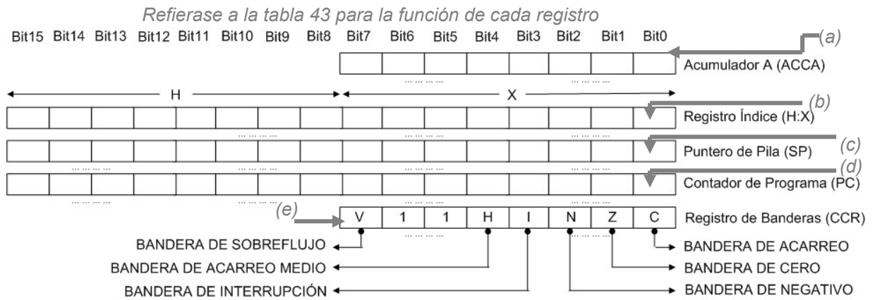
Figura 77. Registros del CPU08. (a) El registro A es un registro usado para operaciones lógicas y aritméticas. (b) El registro H:X comunmente se utiliza para moverse alrededor de la memoria. (c) El SP contiene la dirección del posible siguiente dato a almacenarse en la pila. (d) El PC contiene la siguiente dirección de la instrucción a usarse. (e) El CCR indica el resultado de las operaciones efectuadas por el CPU.
