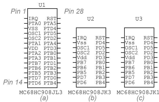
Figura 75. Esquemáticos de los Encapsulados de los Microcontroladores de la Familia HC08 de Motorola. Microcontrolador: (a) 68HC908JL3 (28 pines). (b) 68HC908JK3 (20 pines). (c) 68HC908JK1 (20 pines).
